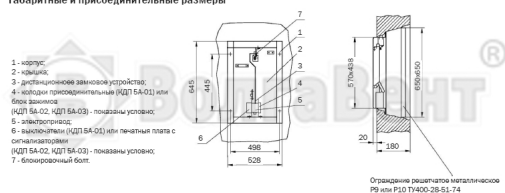
Габаритные и присоединительные размеры
